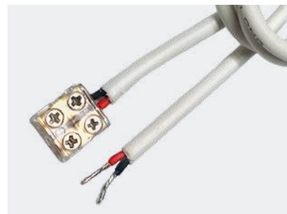
TL-EXT6FT-2-10 Connecteur fileté à 2 épingles - Extension de 6 pieds
